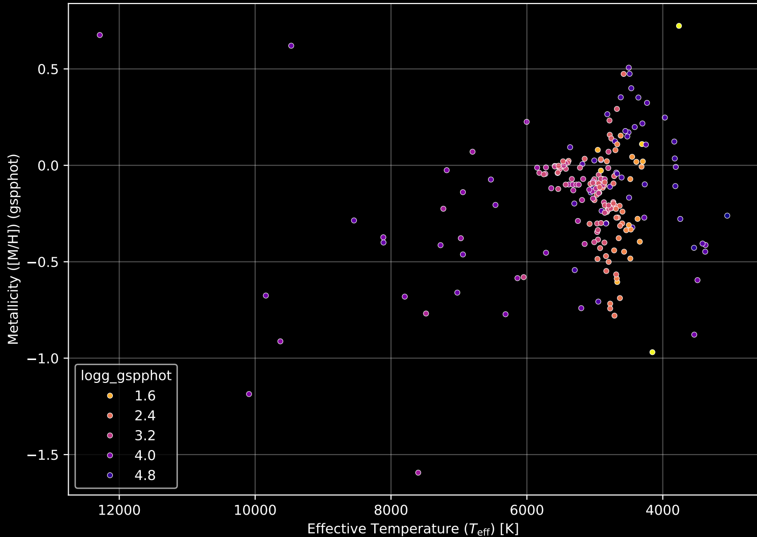
APOGEE DR17 Field: [N2243-S] Stellar Population Parameters (n= 213)
